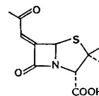
Ro 15-1903 ( 8n )
