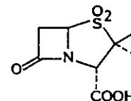
Sulbactam ( 3 )
